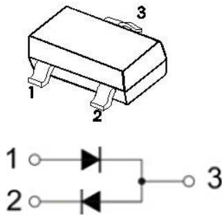
SOT-23
